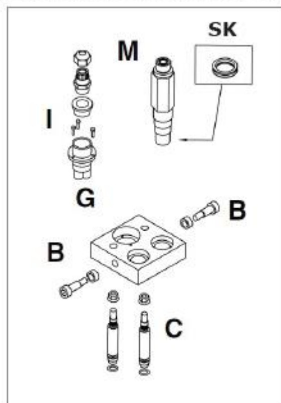
Mobile Half / Parte Móvel / Placa móvil / Partie Mobile
