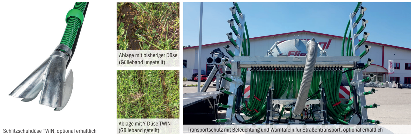
Schlitzschuhdüse TWIN, optional erhältlich
