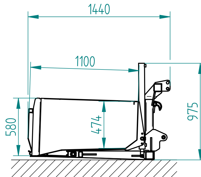
Schnitt A-A
